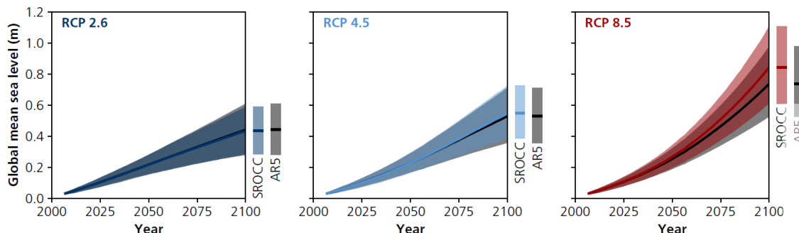
Figura 12. Series temporales de la media mundial del nivel del mar para los RCP 2,6, RCP 4,5 y RCP 8,5, tal y como se estiman en el informe especial del IPCC (2019)7 y, para referencia, los resultados del AR5
