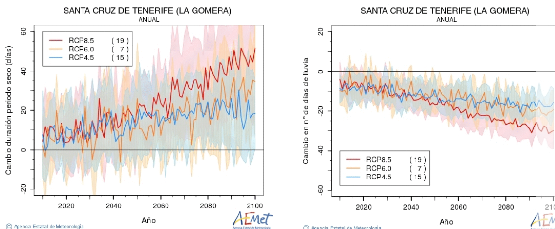
Figura 10. Cambio en la duración del periodo seco y cambio en el número de días de lluvia previstos para La Gomera. Técnica estadística de regresión.
