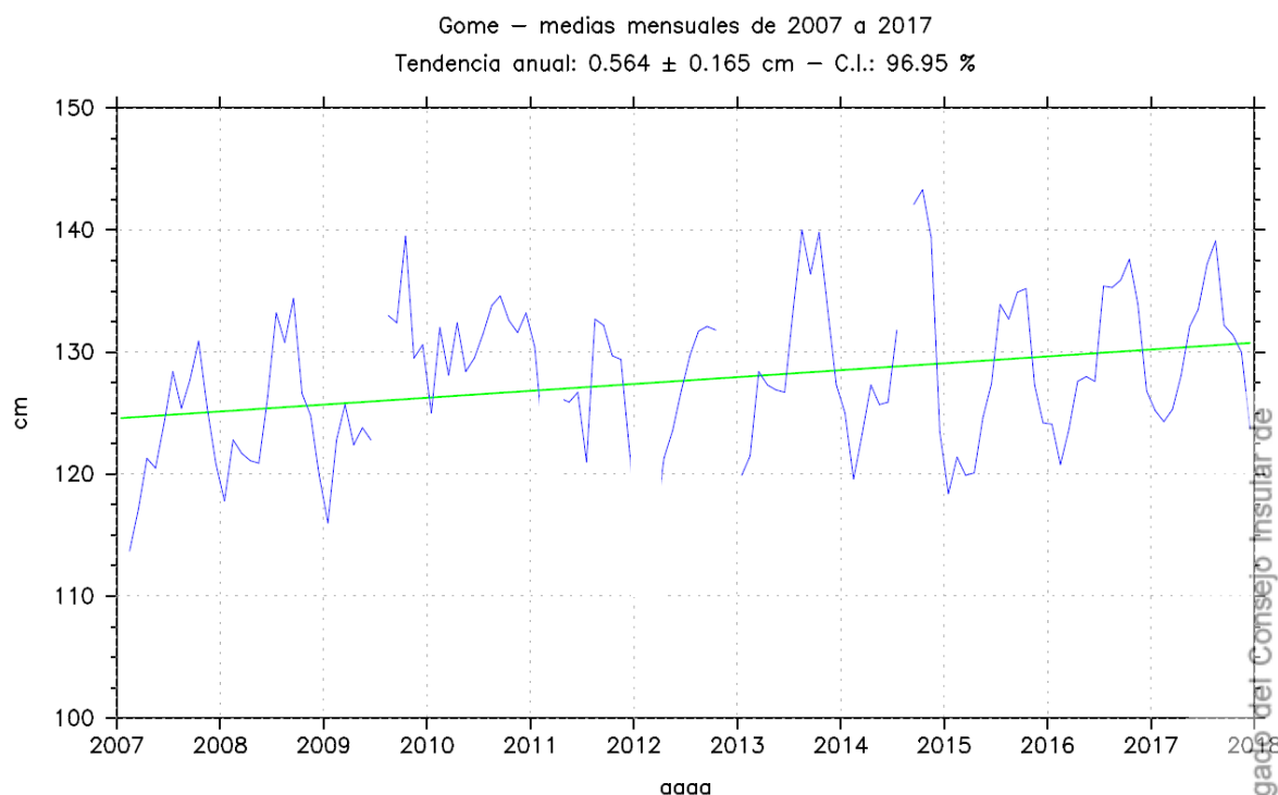
Figura 13. Serie de nivel medio mensual (cm) del mar para el mareógrafo de REDMAR del puerto de San Sebastián de La Gomera. La unidad del nivel medio del mar es el cm.
