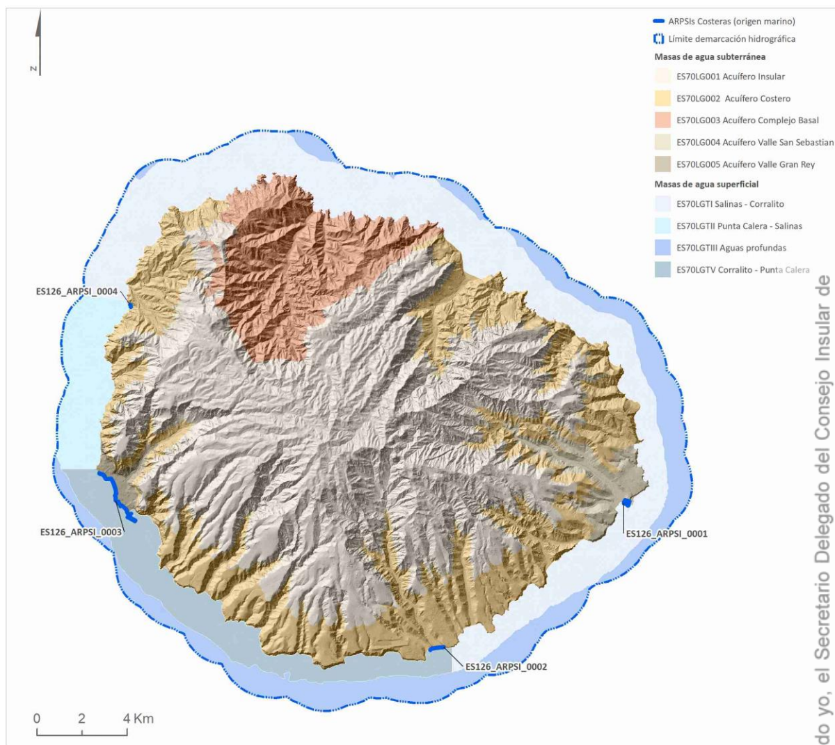
Figura 4. ARPSIs de origen costero
