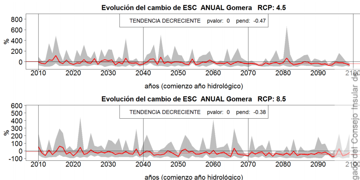
Figura 11. Evolución de la Escorrentía Anual en La Gomera para RCP 4,5 y RCP 8,5.
