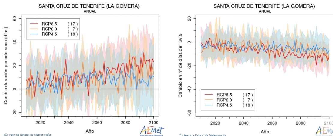
Figura 9. Cambio en la duración del periodo seco y cambio en el número de días de lluvia previstos para La Gomera. Técnica estadística de análogos.
