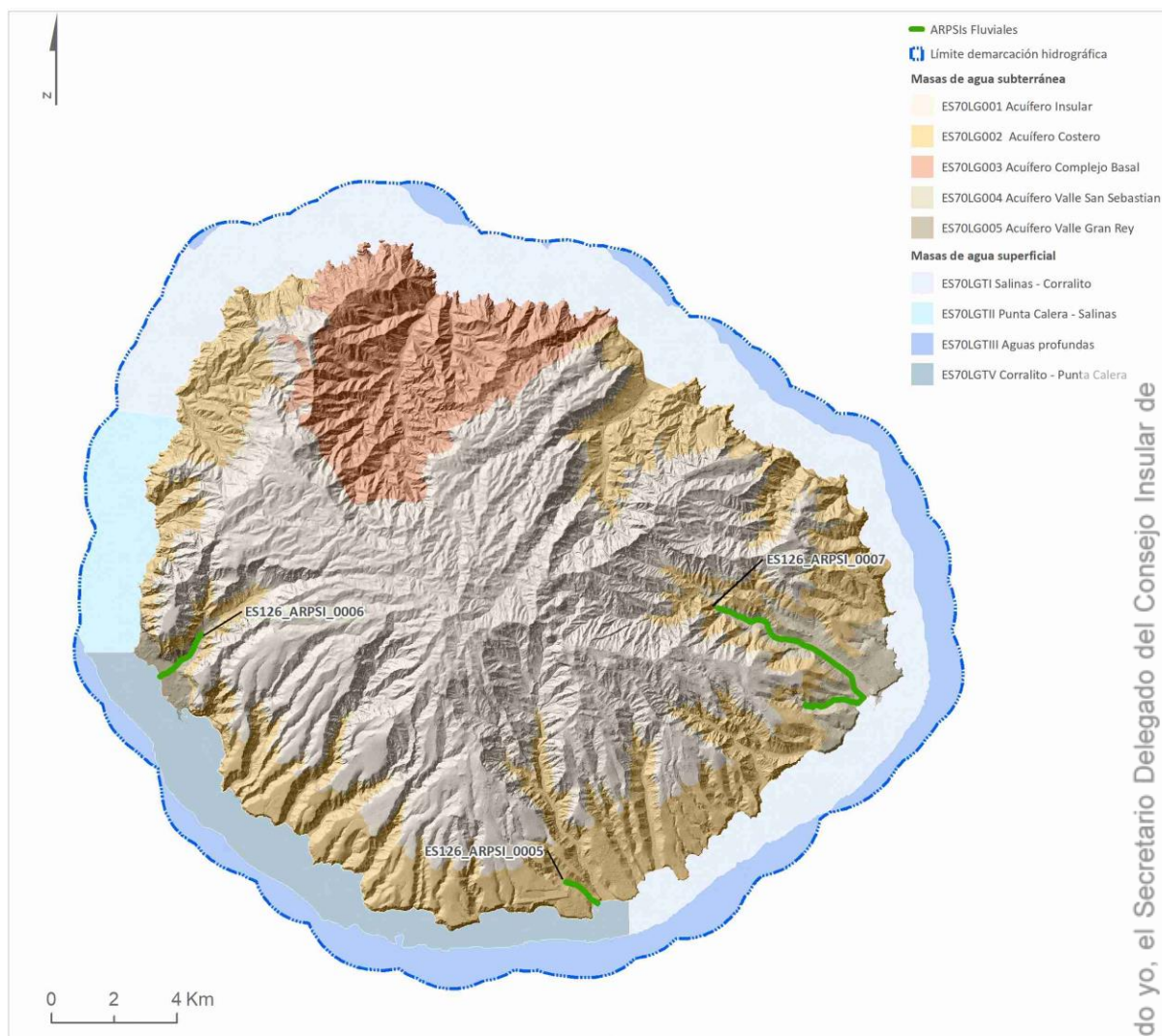
Figura 3. Situación de las ARPSIs de origen fluvial-pluvial
