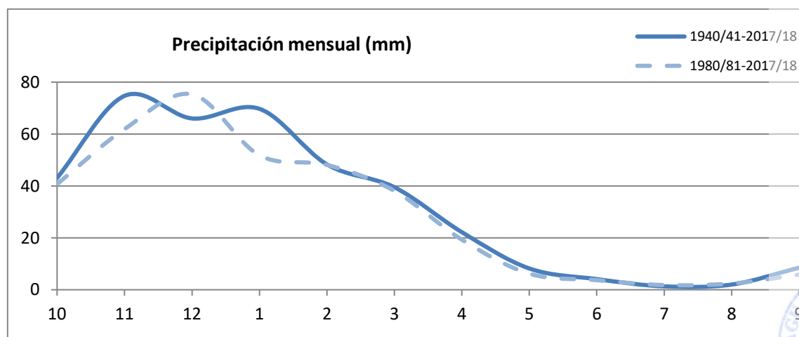
Figura 7. Serie de promedios mensuales de precipitación en La Gomera, 1940/41-2017/18 y 1980/81-2017/18 (CEDEX, 2020) 10
