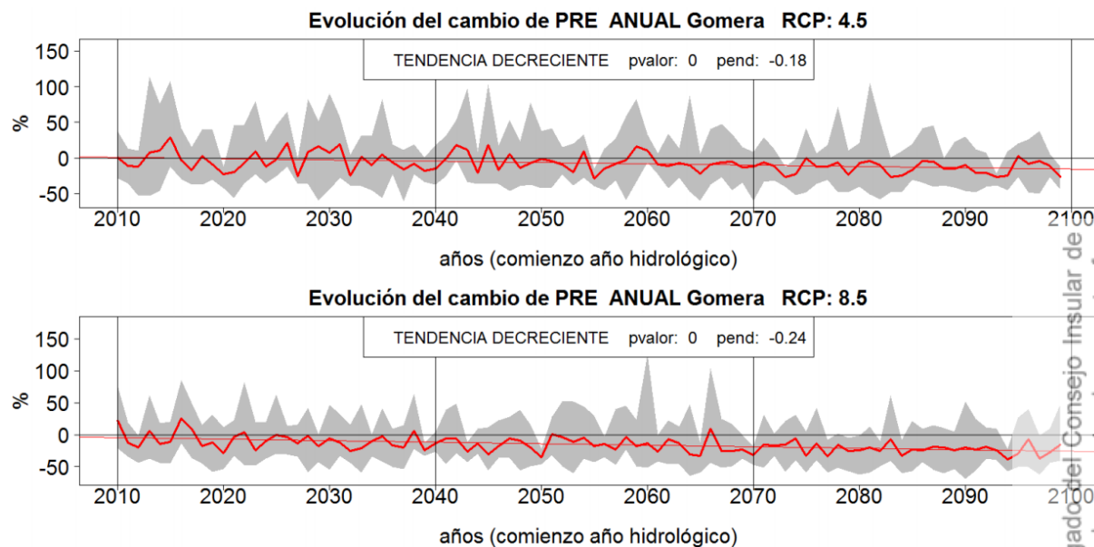
Figura 8. Evolución de la Precipitación Anual en La Gomera para RCP 4,5 y RCP 8,5.
