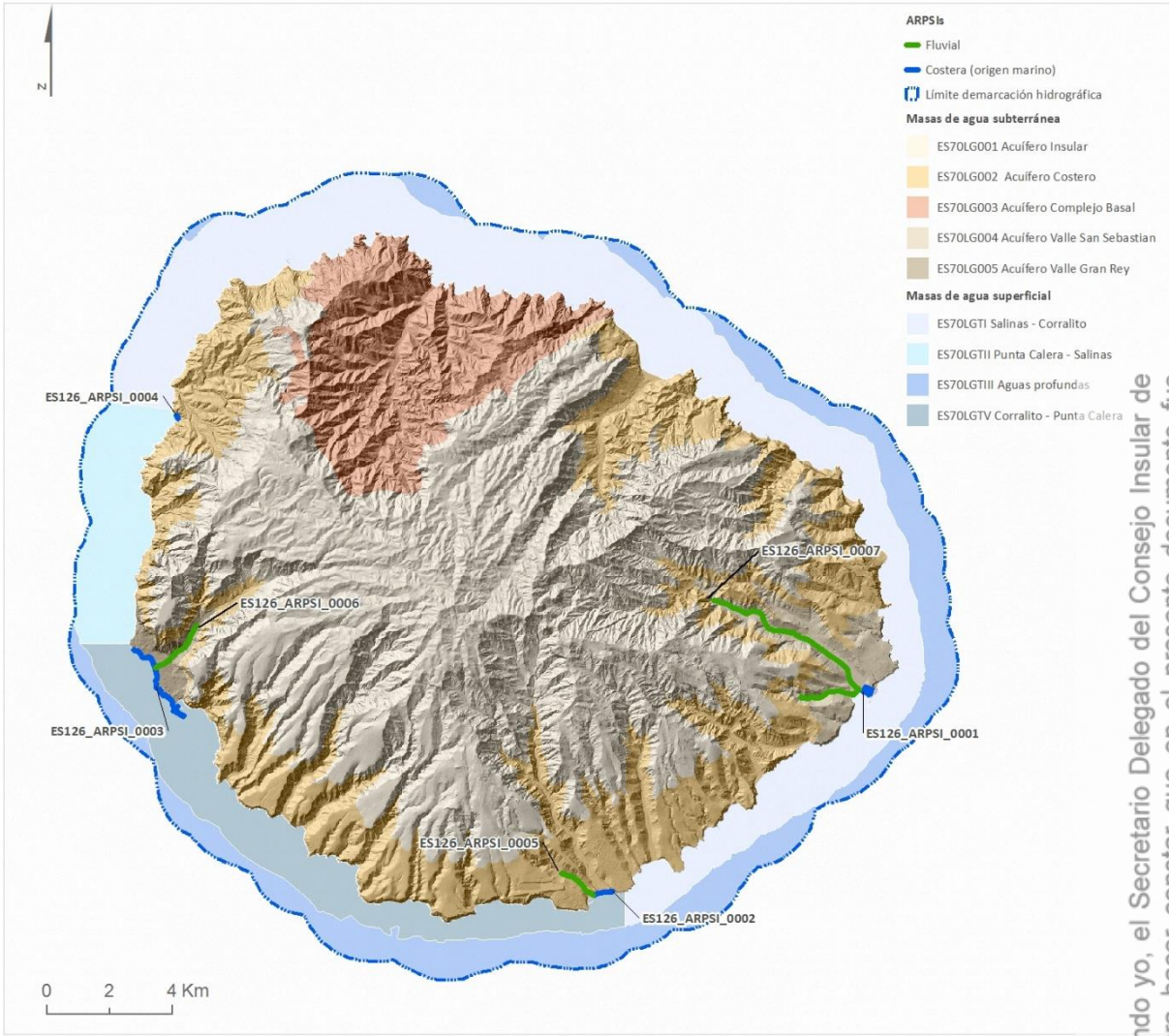
Figura 14. Relación espacial entre masas de agua y ARPSIs de la DHLG
